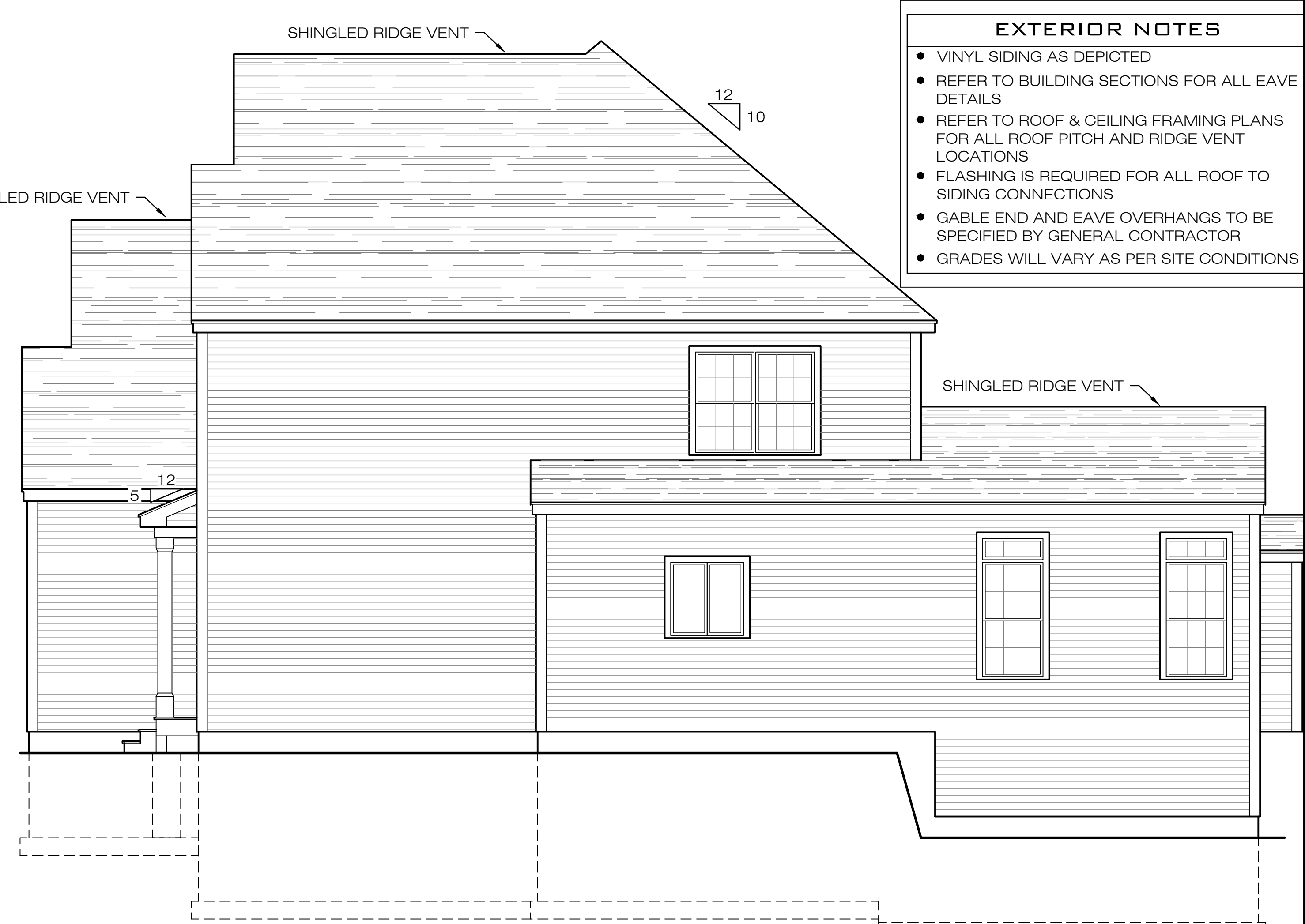
RIGHT ELEVATION
